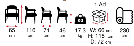
PASS [PSS 07] Şef
