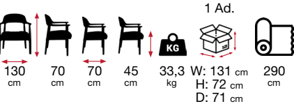
CEMRE [ CMR 02] Tekli
