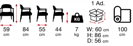
MAKO [ MKO 05] Tel Ayak
