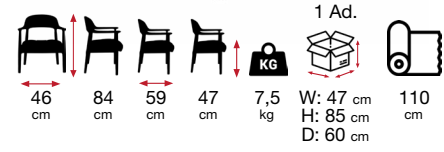
ERA [ ERA 03 ] Ahşap
